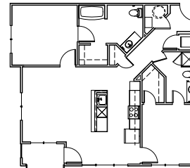
10 B2-4 UNIT PLAN - 1070 SF SCALE: 1/8" = 1'-0"
