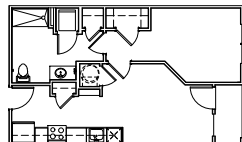
2 B1-1 UNIT PLAN - 573 SF SCALE: 1/8" = 1'-0"
