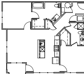
7 B2-1 UNIT PLAN - 1070 SF SCALE: 1/8" = 1'-0"
