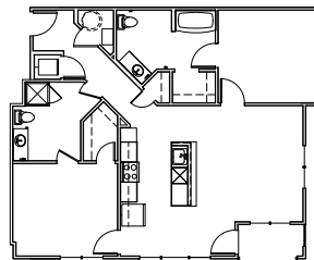
12 B2-6 UNIT PLAN - 1120 SF SCALE: 1/8" = 1'-0"
