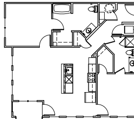
9 B2-3 UNIT PLAN - 1070 SF SCALE: 1/8" = 1'-0"
