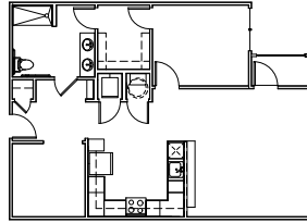
5.1 B1-4.1 UNIT PLAN - 958 SF SCALE: 1/8" = 1'-0"
