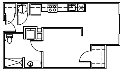
1 S-1 UNIT PLAN - 549 SF SCALE: 1/8" = 1'-0"
