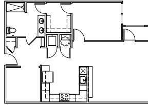
5 B1-4 UNIT PLAN - 969 SF SCALE: 1/8" = 1'-0"
