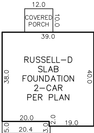
INSET N.T.S.
