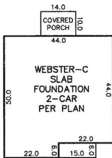
INSET N.T.S.
