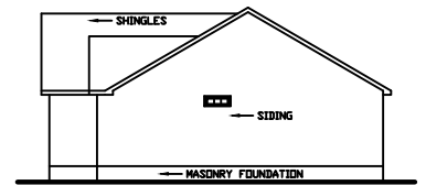
RIGHT ELEVATION
